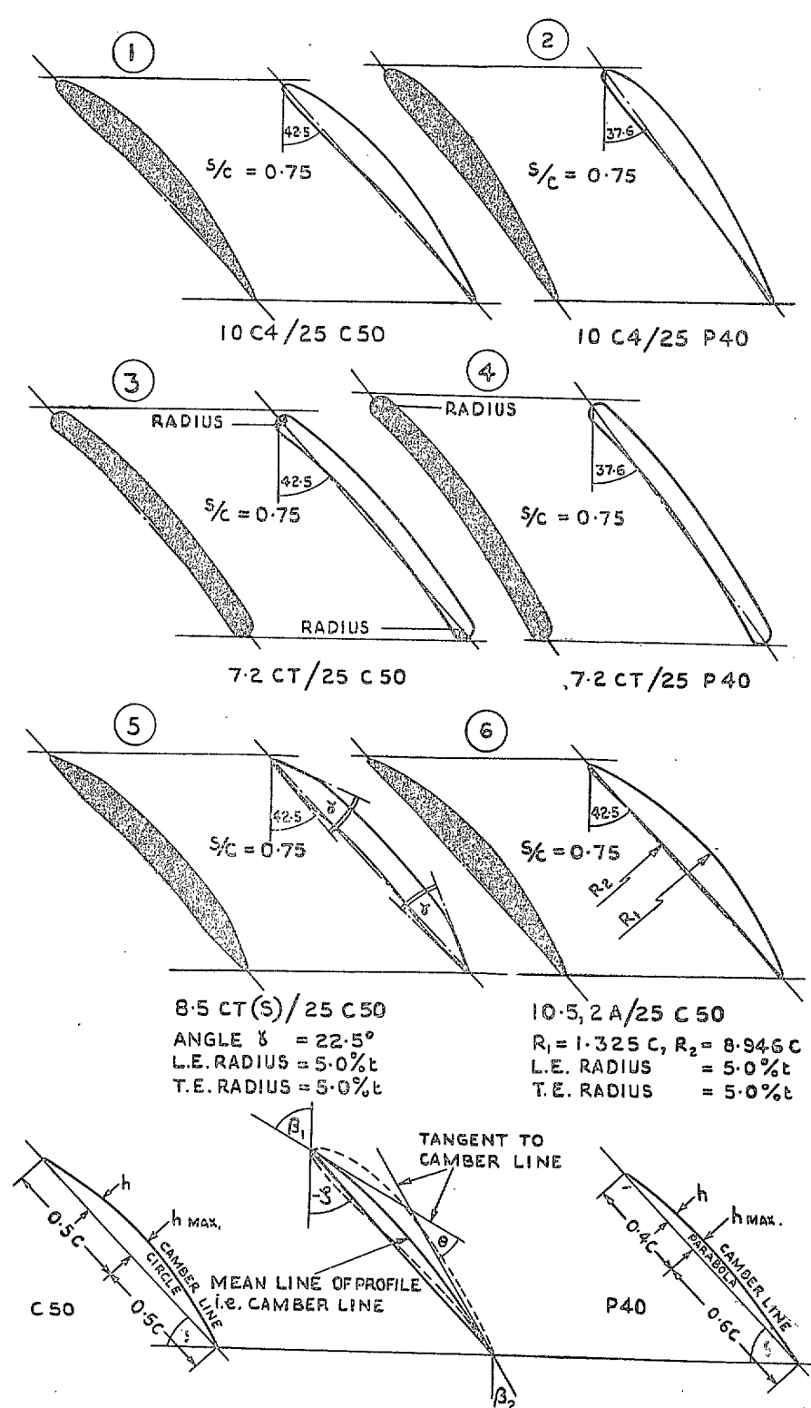
FIG. 2. Cascade data.
