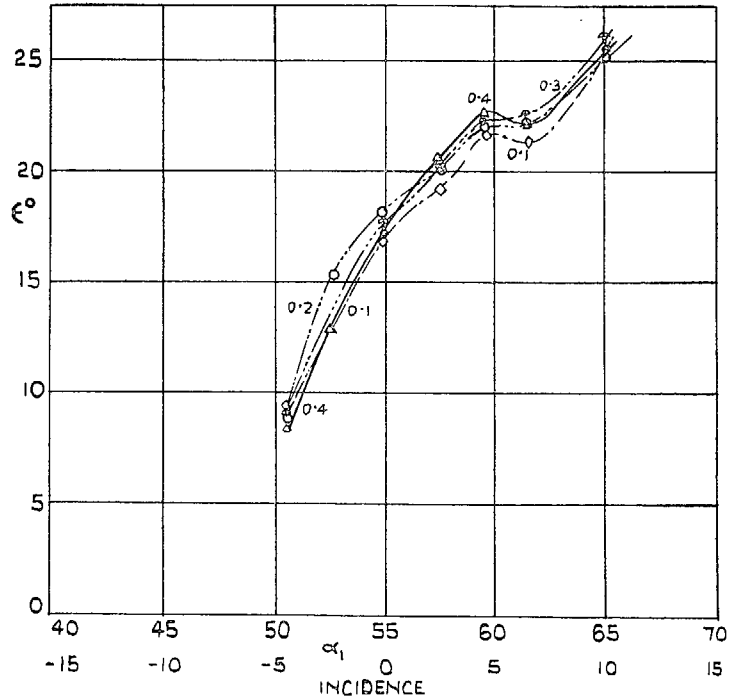
FIG. 7. Cascade 7.2CT/25C50.
