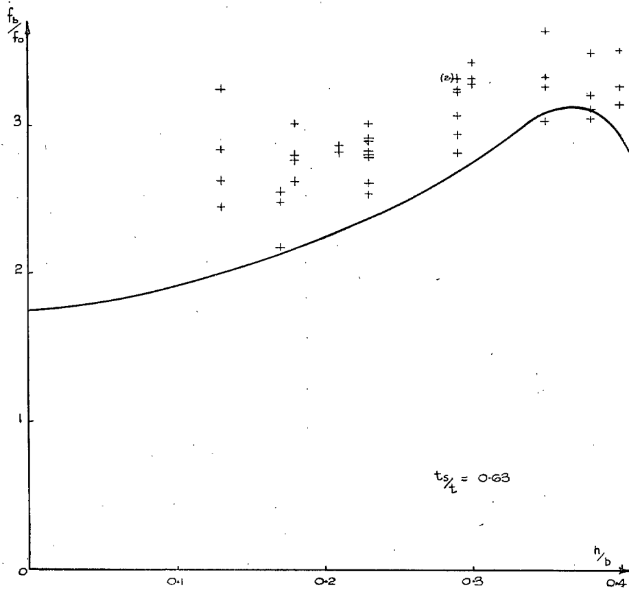
FIG. 9. Comparison with American results (N.A.C.A. T.N.1553).
