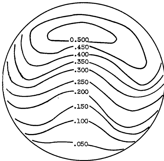
(d) \theta_1, 44.7^\circ ; \alpha, 10^\circ ; cone deflection, 10^\circ ; critical pressure recovery.
