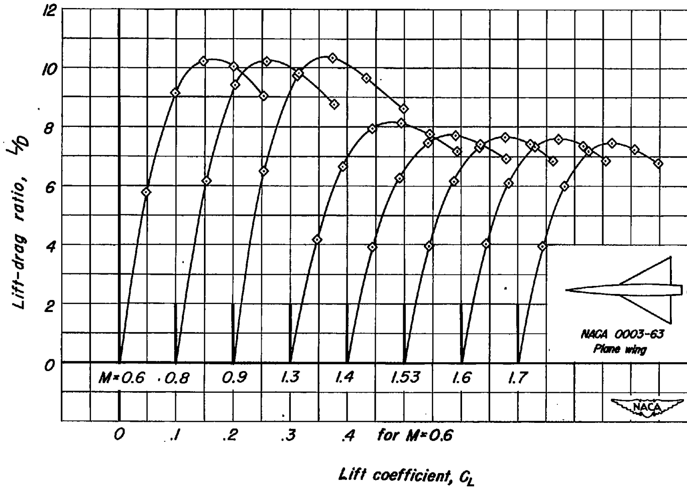
(d) L/D vs C_L
