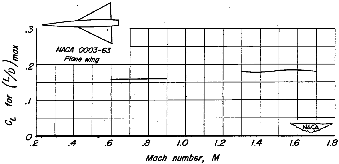
(d) C_L for (L/D)_{max} vs M
