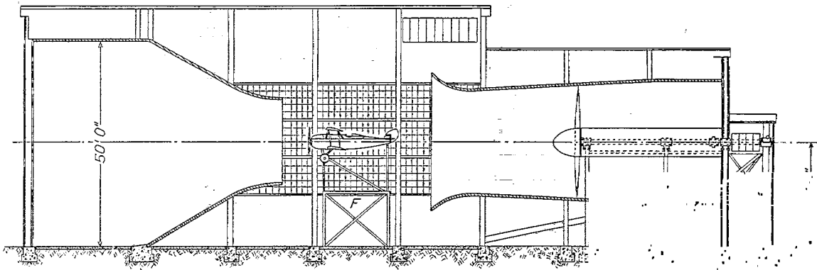
LONGITUDINAL SECTION
